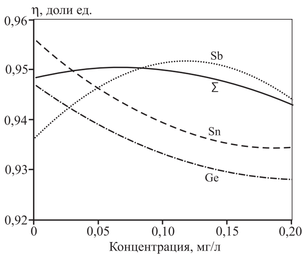
Рис. 1. Зависимость выхода по току цинка ( \eta ) от концентрации примесей — раздельной (Sb, Sn и Ge) и совместной ( \Sigma = \frac{1}{3}Sb + \frac{1}{3}Sn + \frac{1}{3}Ge )
