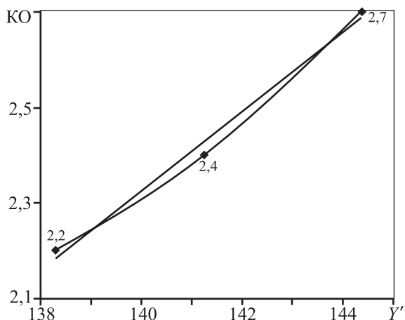
Рис. 2. Зависимость значения яркости электролита от криолитового отношения
