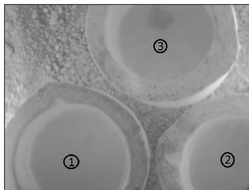
Рис. 1. Состояние поверхности электролита в зависимости от значения криолитового отношения 1 — КО = 2,2 , 2 — 2,4 и 3 — 2,7
