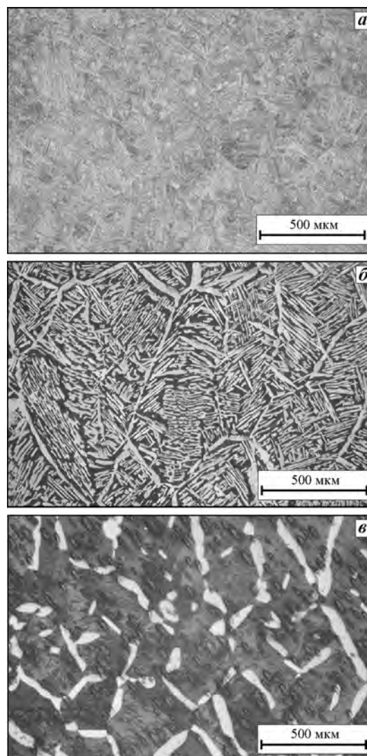
Рис. 2. Оптические микрофотографии сплава Ti—4мас.%Co a — исходный литой; б — отожженный при t = 690 °C ( \tau = 720 ч), в — при 780 °C (780 ч)
