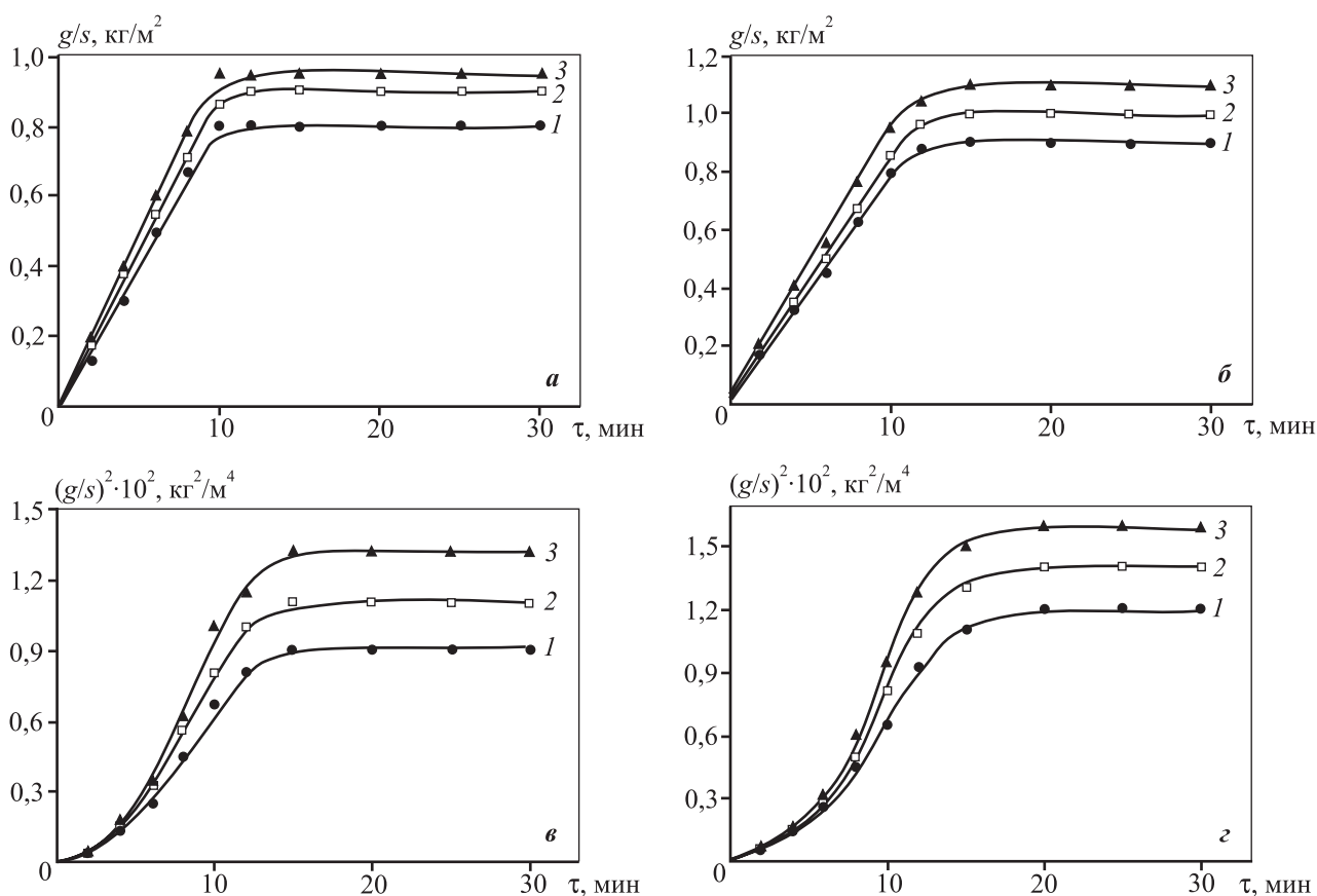
Кинетические кривые окисления сплава АК7М2 + 0,05%Sr без модифицирования (а) и с добавкой Ge в количестве, мас. %: 0,3 (б), 0,6 (в), 1,0 (г) T = 773 \text{ К (1)}, 798 \text{ К (2)} \text{ и } 823 \text{ К (3)}
