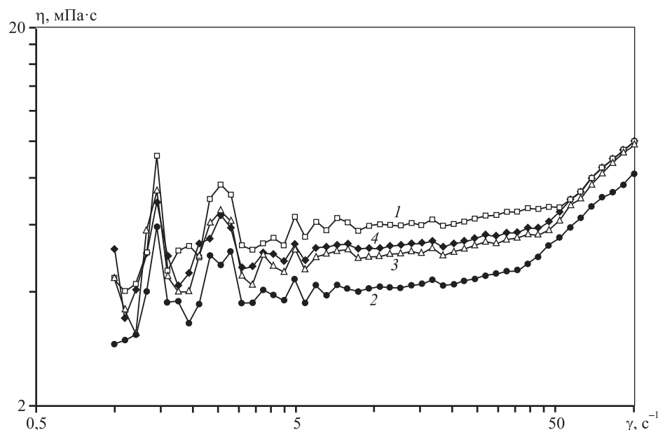
Рис. 3. Кривые вязкости расплавов на основе \text{LiF—BeF}_2 при t = 700 °C
