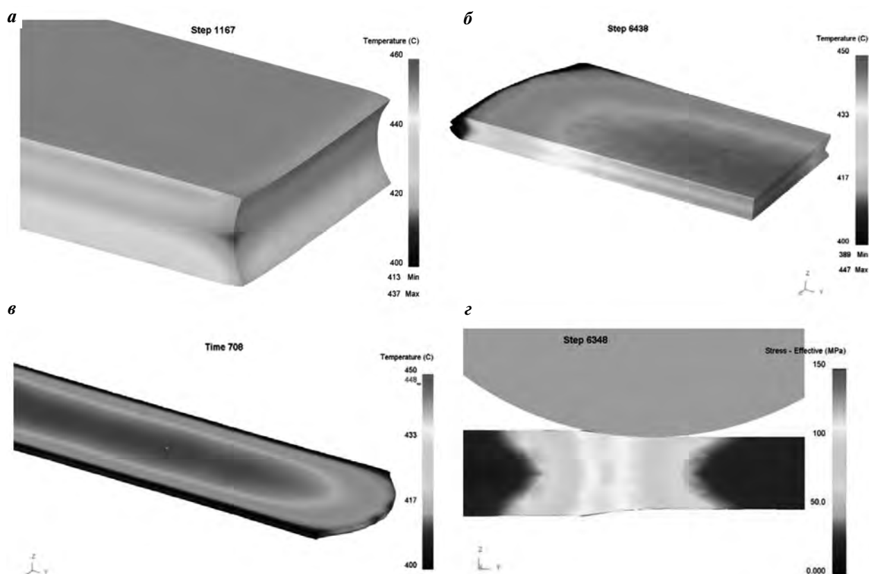
Рис. 1. Распределение температуры на поверхности после 4 (а), 16 (б) и 28 (г) проходов, а также интенсивности напряжений по сечению проката (з)
