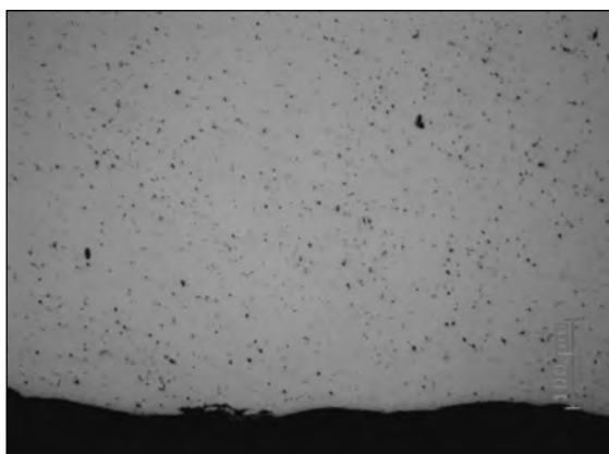
Рис. 4. Микроструктура сварного шва исследуемого сплава после межкристаллитной коррозии ( \times 200 )
