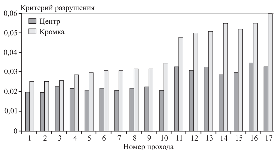
Рис. 2. Значения критерия Кокрофта–Латама по проходам
