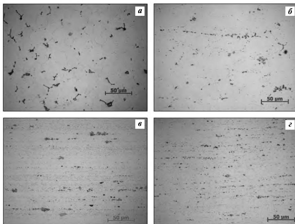
Рис. 3. Микроструктуры полуфабрикатов из опытного сплава в различных состояниях ( \times 500 )
