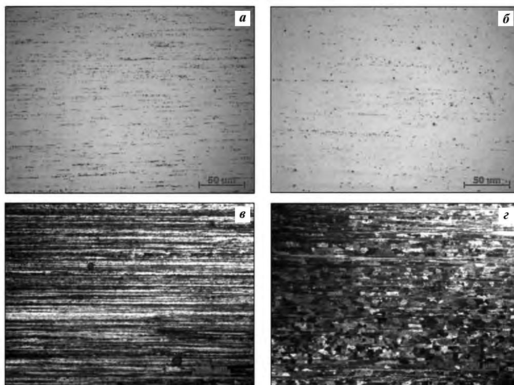
Рис. 5. Микроструктура прутка из опытного сплава диаметром 9 мм ( а ), а также проволоки диаметром 3 мм в деформированном ( б, в ) и отожженном ( з ) состояниях а, б — увеличение 500 \times ; в, з — 200 \times
